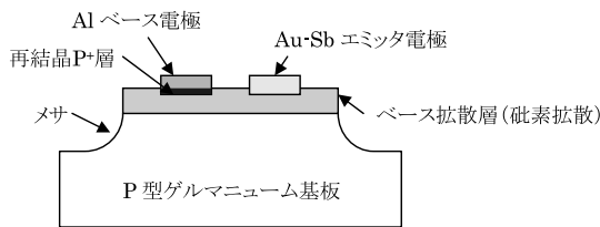
図2 ゲルマニウム拡散ベース トランジスタ
