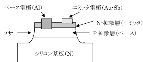
図1 ベル研究所1956年の2重拡散型トランジスタ
